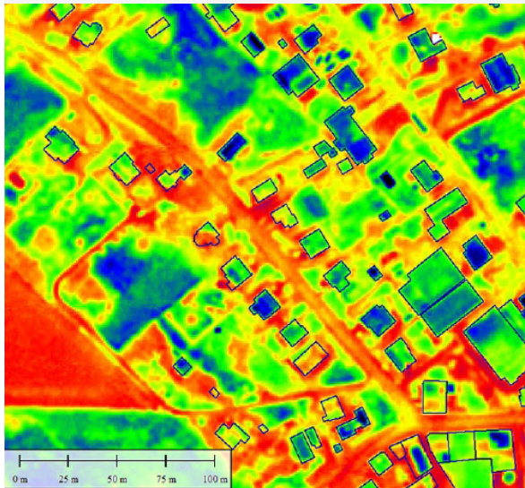
Thermografiebilder, zusammgeführt mit Katasterdaten (Quelle: Hexagon/Miramap)
